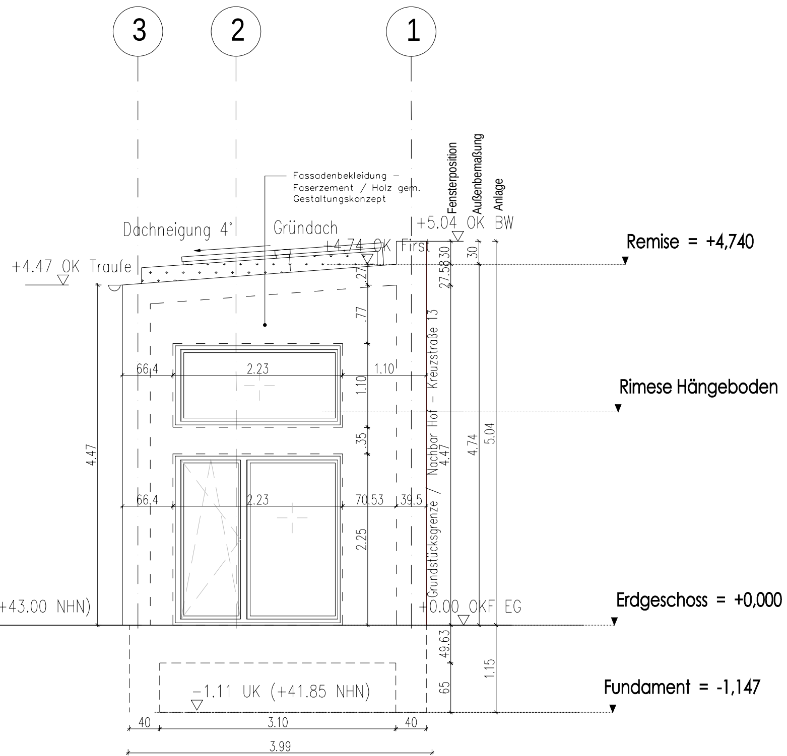
Ansicht B2.3 - Westen
